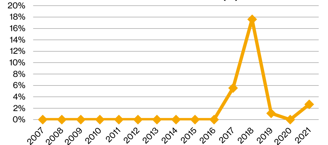
Taux d'autosuffisance (%)
